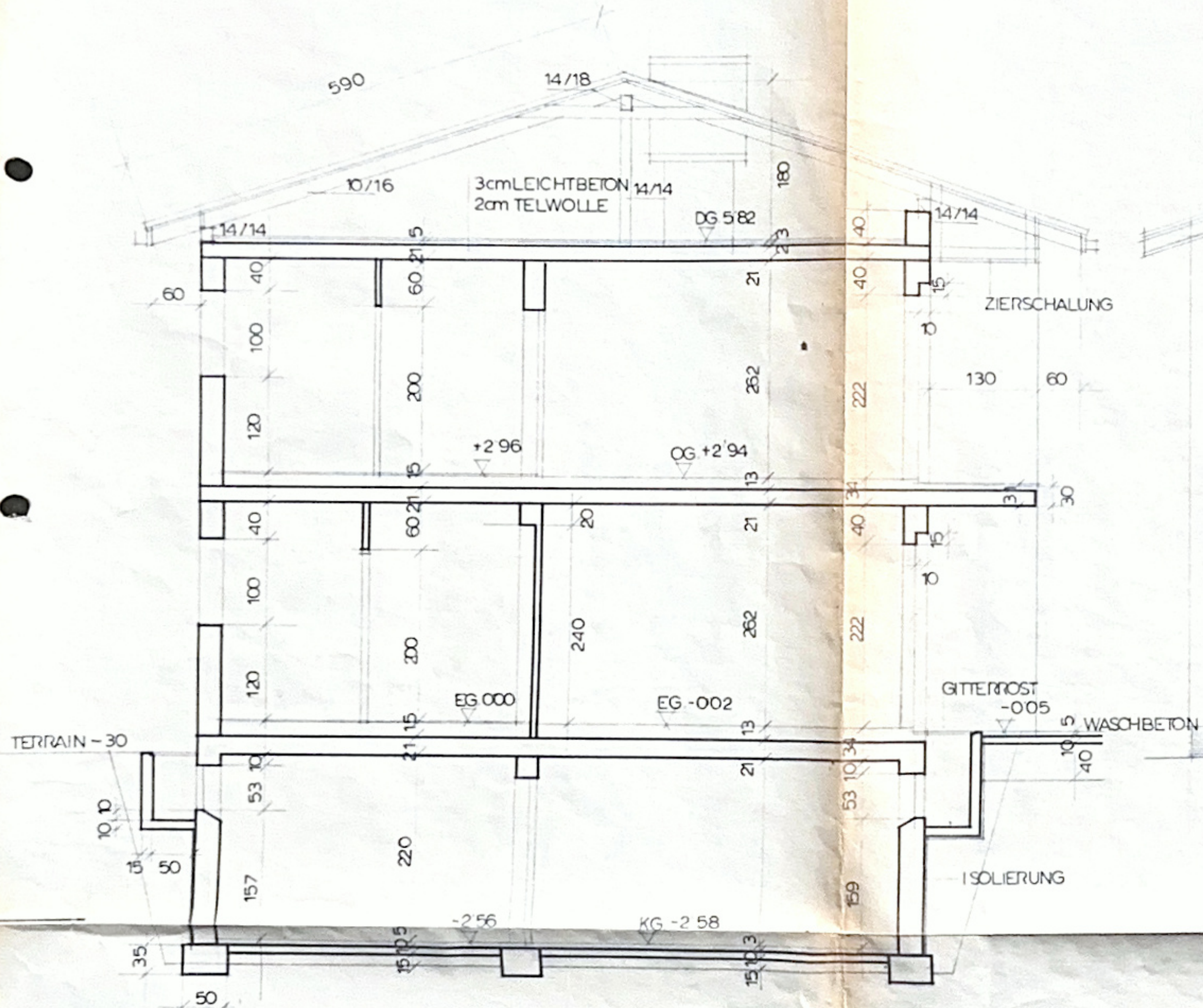
SCHNITT WOHNHAUS
